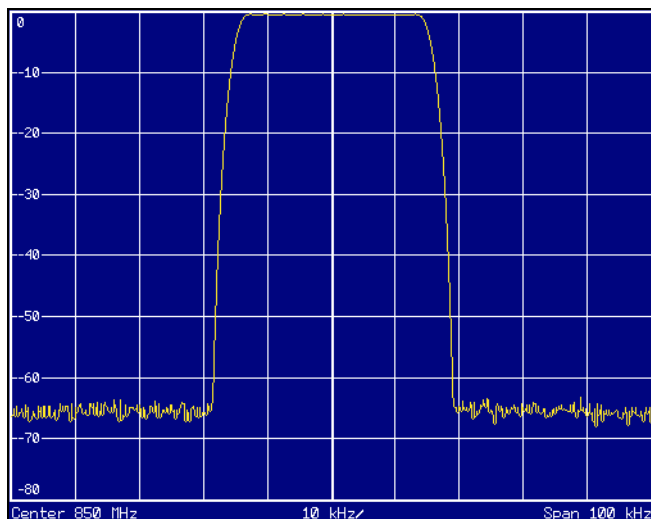
Bild 2-26 Frequenzgang des 30-kHz-Kanalfilters zur Messung der Leistung im IS 95-Nachbarkanal
