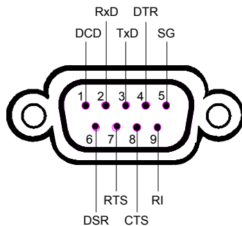
Bild 8-4 Pinbelegung der RS-232-Schnittstelle
