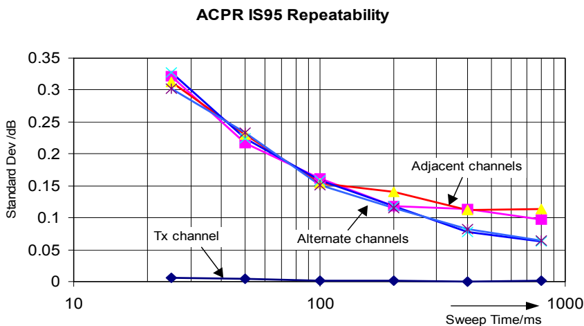
Bild 2-25 Wiederholgenauigkeit der Nachbarkanalleistungsmessung in der Fast-ACP-Betriebsart bei Signalen nach dem IS95-Standard
