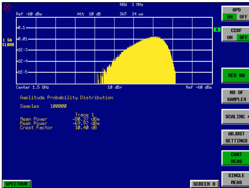
Bild 2-35 Darstellung der Amplituden-Wahrscheinlichkeitsverteilung von weißem Rauschen
