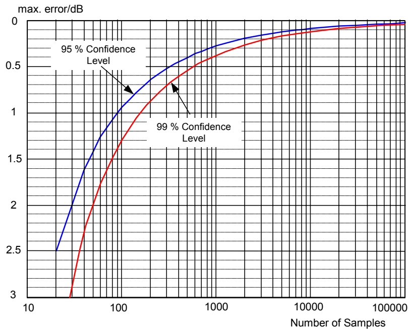
Bild 2-16 Wiederholgenauigkeit der Kanalleistungsmessung abhängig von der Anzahl der Samples zur Berechnung der Leistung
