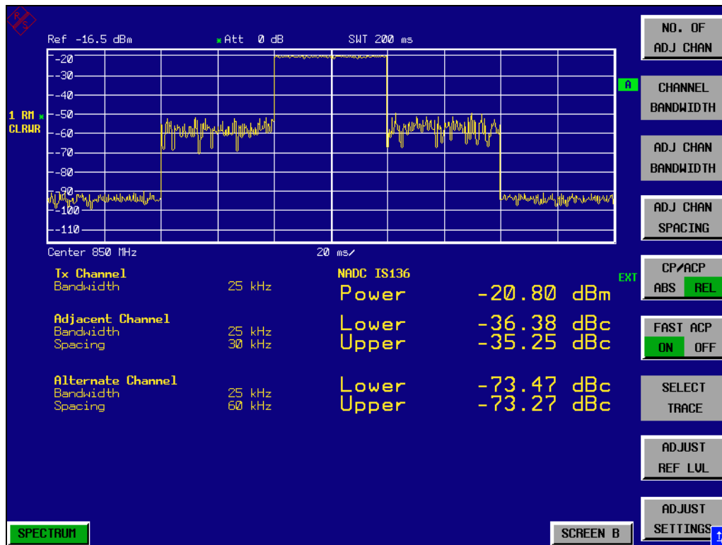
Bild 2-28 Messung der Nachbarkanalleistung im Zeitbereich (Fast ACP)
