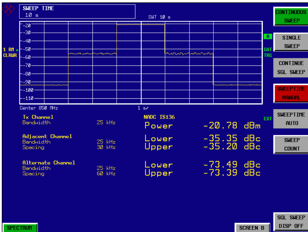
Bild 2-31 Darstellung der Nachbarkanalleistung die durch das Modulationsspektrum und das Transientspektrum entsteht.
