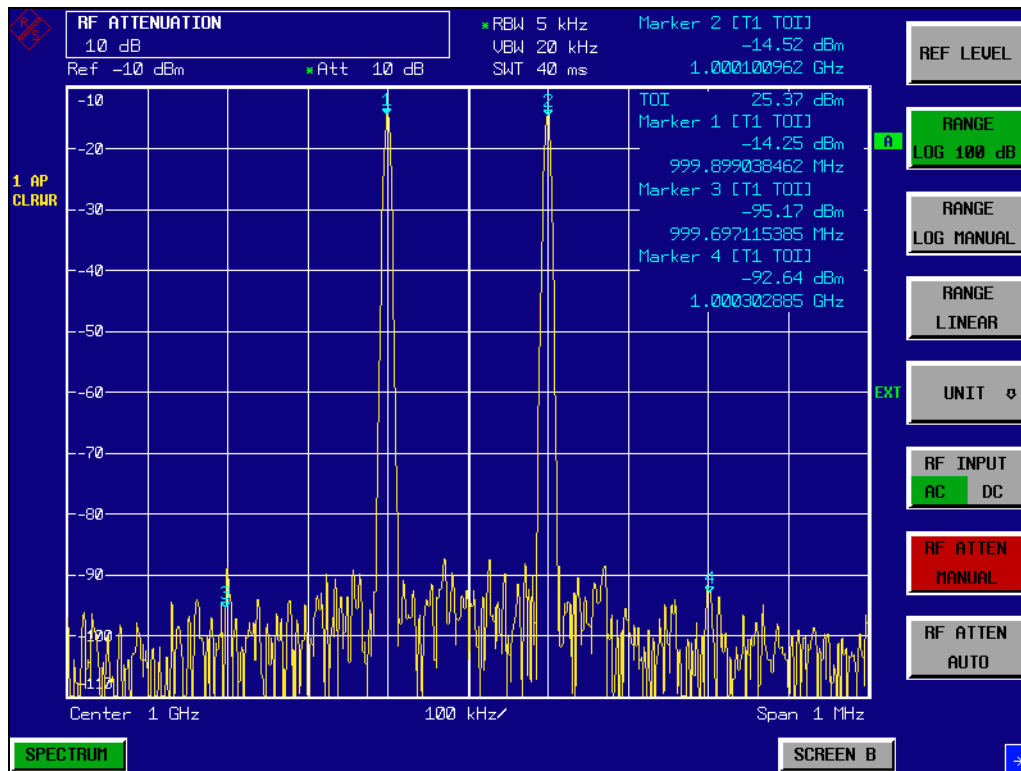
Bild 2-4 Durch Erhöhung der HF-Dämpfung verschwinden die R&S FSQ.-Eigenstörprodukte im Rauschen.
