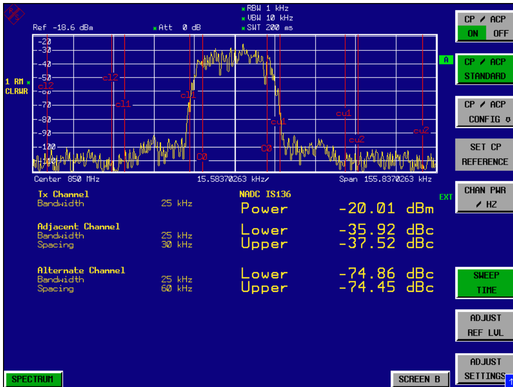
Bild 2-27 Messung der relativen Nachbarkanalleistung eines NADC-Signals in je zwei Nachbarkanälen unterhalb und oberhalb des Sendekanals.
