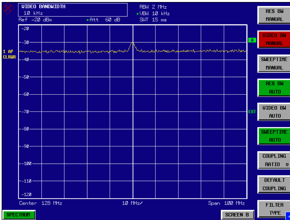
Bild 2-11 Darstellung eines HF-Sinussignals mit geringem Rauschabstand bei kleiner Videobandbreite.
