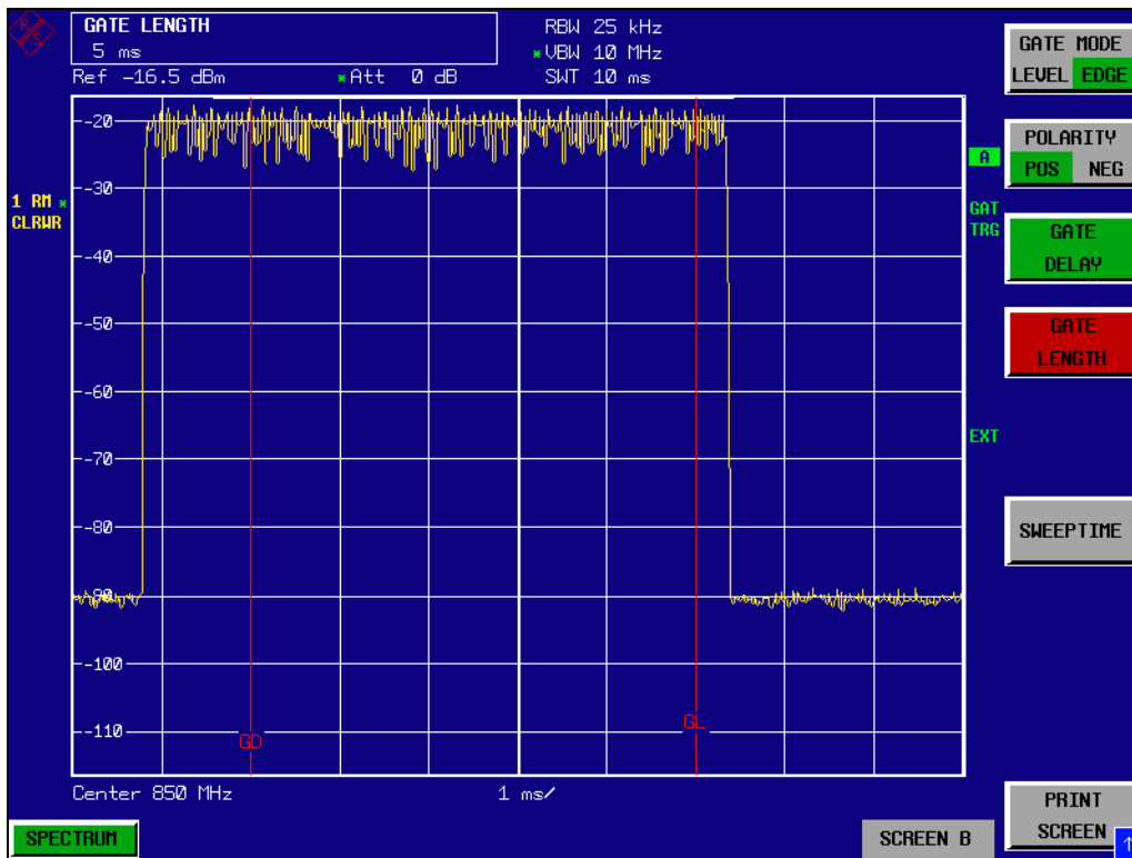
Bild 2-30 Einstellung der Parameter Gate Delay und Gate Length im Zeitbereich. Der Zeitraum, in dem das Spektrum gemessen wird, wird durch zwei senkrechte Linien dargestellt.
