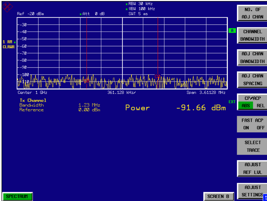
Bild 2-14 Messung der R&S FSQ-Eigenrauschleistung in 1,23 MHz Kanalbandbreite.
