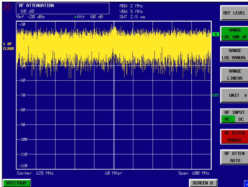
Bild 2-9 Darstellung eines Sinussignals mit kleinem Rauschabstand. Das Signal wird mit dem Auto-Peak-Detektor gemessen fast vollständig durch das Eigenrauschen des Signalanalysators überdeckt.
