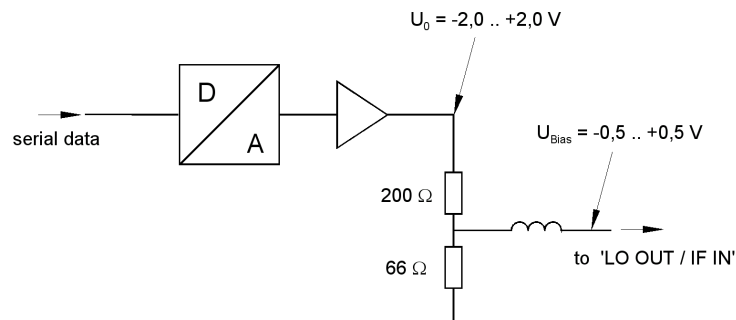
Bild 4-34 Bias-Schaltung des Signalanalysators
