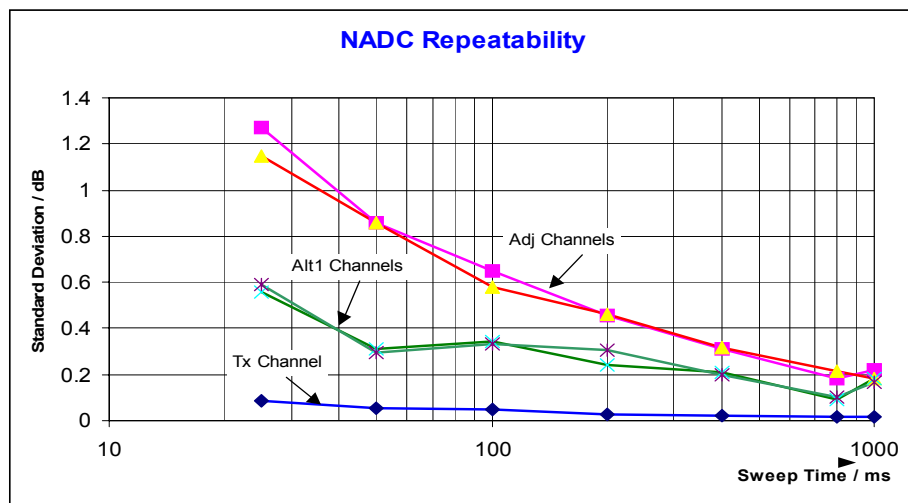
Bild 2-29 Standardabweichung des Messergebnisses bei der Fast-Ach-Messung in Abhängigkeit von der gewählten Sweepzeit ermittelt aus jeweils 100 Messungen pro Sweepzeit.
