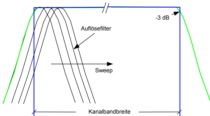
Bild 2-15 Approximation des Kanalfilters durch Sweepon mit kleiner Auflösungsbandbreite
