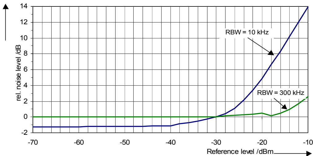
Bild 2-7 Änderung des angezeigten Rauschens abhängig vom eingestellten Referenzpegel bei 10 kHz und 300 kHz Bandbreite (Bezug = -30 dBm Referenzpegel)
