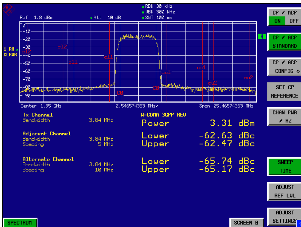
Bild 2-32 Messung der relativen Nachbarkanalleistung an einem W-CDMA-Uplink-Signal.
