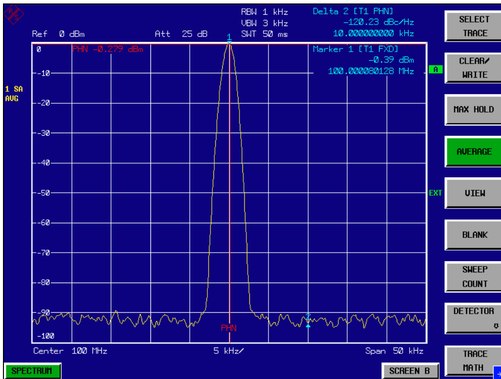
Bild 2-17 Messung des Phasenrauschens mit der Marker-Funktion Phase Noise
