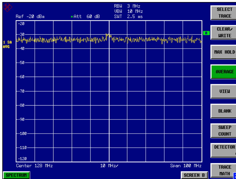
Bild 2-10 Darstellung eines HF-Sinussignals mit geringem Rauschabstand bei Mittelung der Messkurve.
