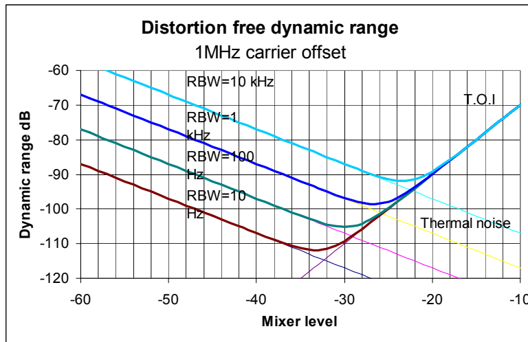
Bild 2-5 Intermodulationsfreier Bereich des R&S FSQ abhängig vom Pegel am Eingangsmischer und der eingestellten Auflösungsbreite (Nutzsignalabstand = 1 MHz, DANL = -157 dBm /Hz, T.O.I = 25 dBm; typ. Werte bei 2 GHz)
