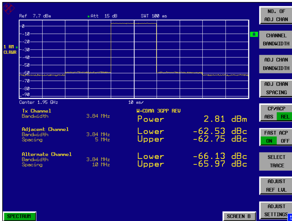
Bild 2-33 Messung der Nachbarkanalleistung eines W-CDMA-Signals mit der Fast-ACP-Methode.
