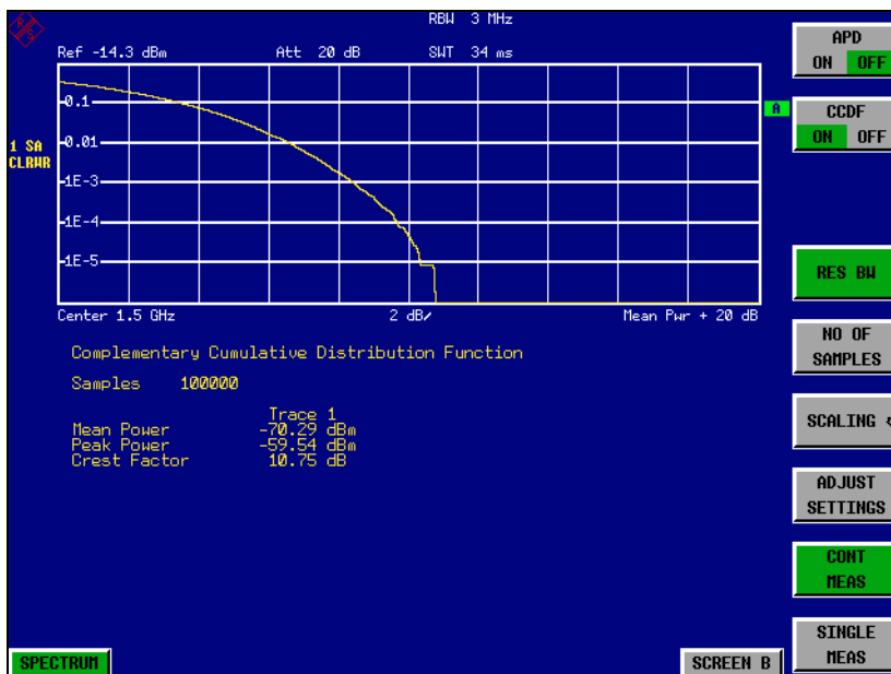
Bild 2-36 Darstellung der CCDF von weißem Rauschen
