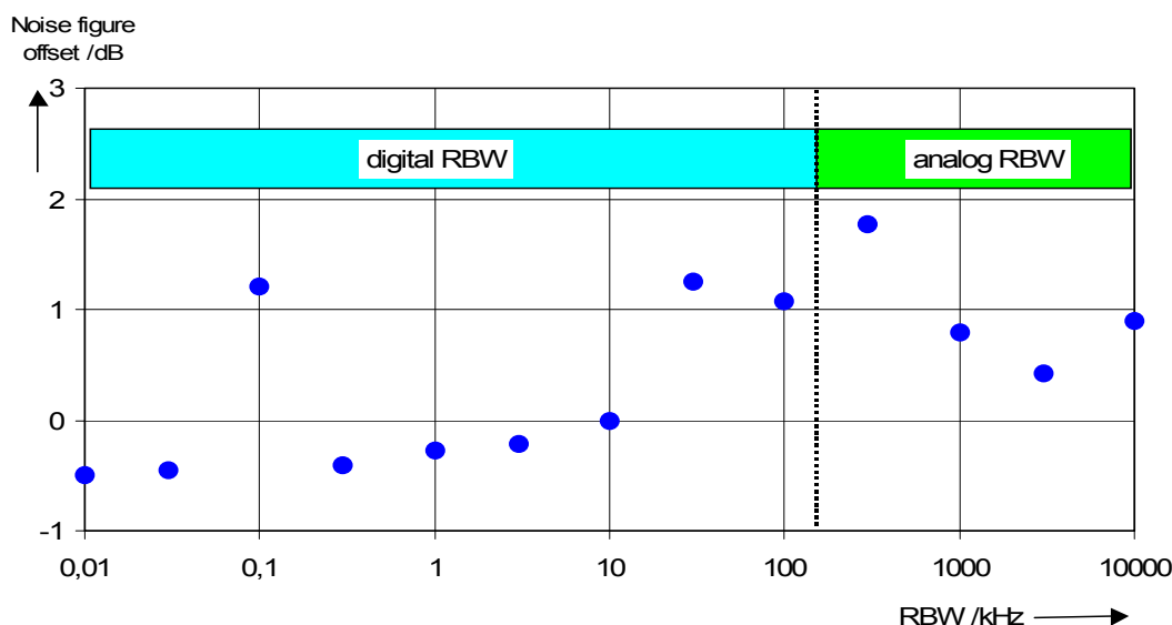
Bild 2-8 Änderung des Rauschmaßes des R&S FSQ bei den verschiedenen Bandbreiten. Als Bezugsbandbreite ist 10 kHz gewählt.
