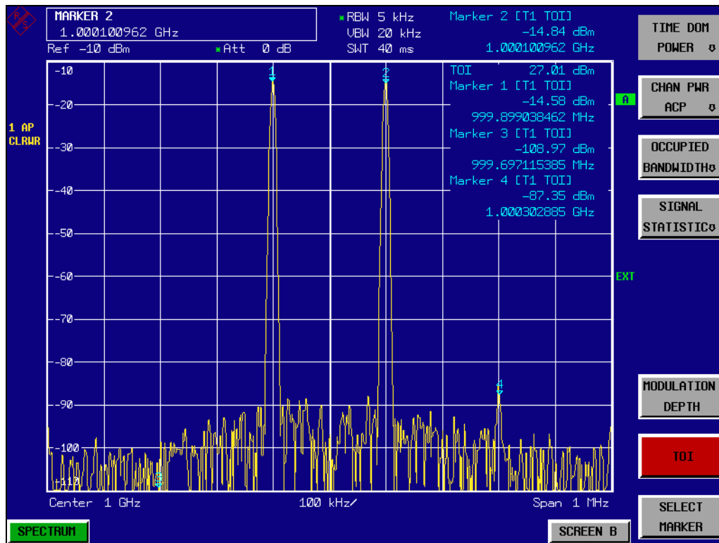
Bild 2-3 Ergebnis der Messung des Eigen-Intermodulationsabstandes des R&S FSQ. Der Interceptpunkt dritter Ordnung (TOI) wird am rechten oberen Rand des Grids ausgegeben
