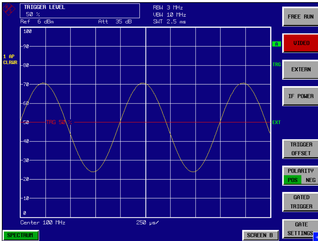
Bild 2-18 Messung des NF-Signals eines mit 1 kHz AM-modulierten Trägers Mit dem AM/FM-Demodulator im R&S FSQ, kann die NF mit einem Lautsprecher abgehört werden.
