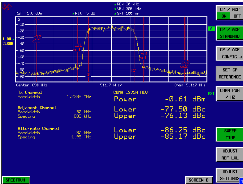
Bild 2-22 Nachbarkanalleistungsmessung an einem CDMA IS95-Signal
