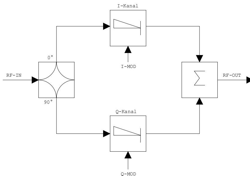
Bild 4-25 I/Q-Modulation
