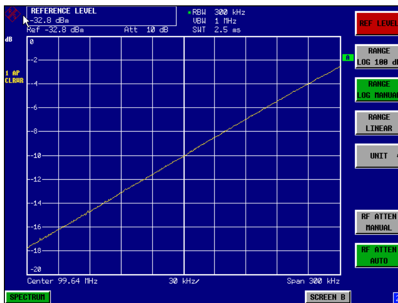
Bild 2-20 Darstellung der Filterflanke des 300-kHz-Filters als FM-Diskriminatorkennlinie.
