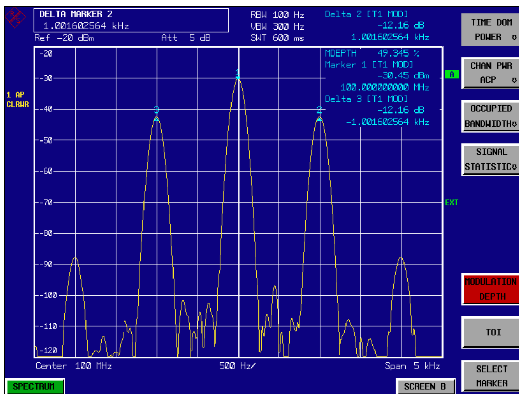
Bild 2-19 Messung des AM-Modulationsgrades. Der Modulationsgrad kann hier mit MDEPTH = 49.345 % abgelesen werden. Die Frequenz des NF-Signals kann der Frequenzanzeige der Delta-Marker entnommen werden
