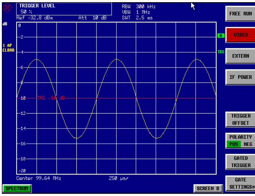
Bild 2-21 Darstellung des demodulierten FM-Signals
