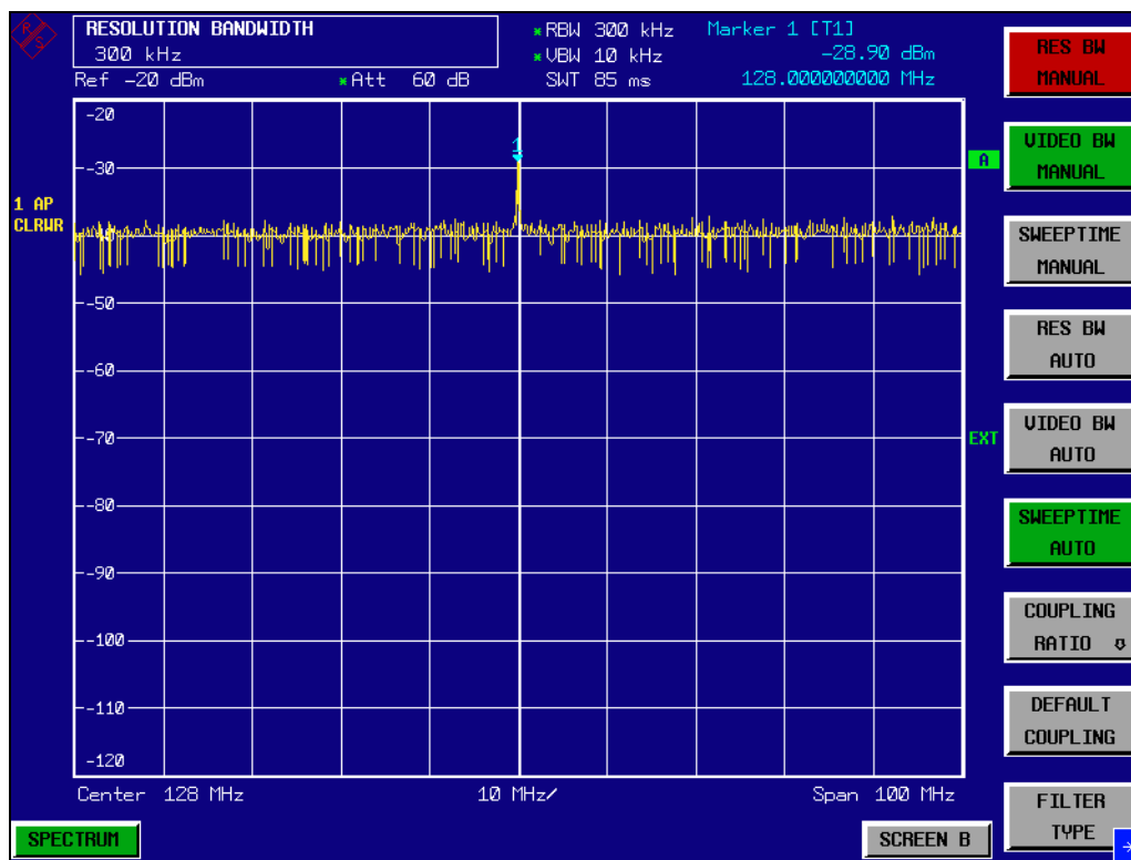
Bild 2-12 Anzeige des Referenzsignals bei kleinerer Auflösebandbreite.
