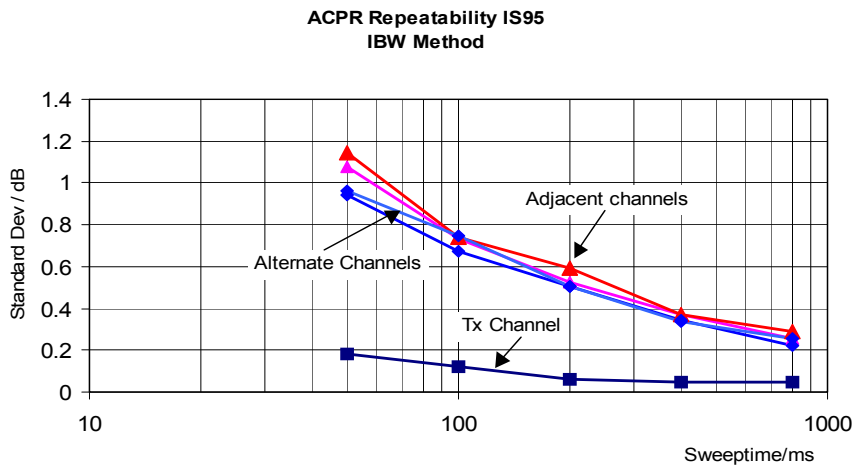
Bild 2-23 Wiederholgenauigkeit der Nachbarkanalleistungsmessung bei Messung nach der Integrationsmethode an Signalen nach dem IS95-Standard.
