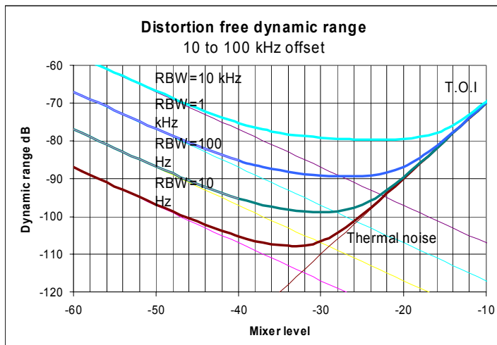
Bild 2-6 Intermodulationsfreier Bereich des R&S FSQ abhängig vom Pegel am Eingangsmischer und der eingestellten Auflösungsbreite (Nutzsignalabstand = 10 bis 100 kHz, DANL = -157 dBm /Hz, T.O.I = 25 dBm; typ. Werte bei 2 GHz)
