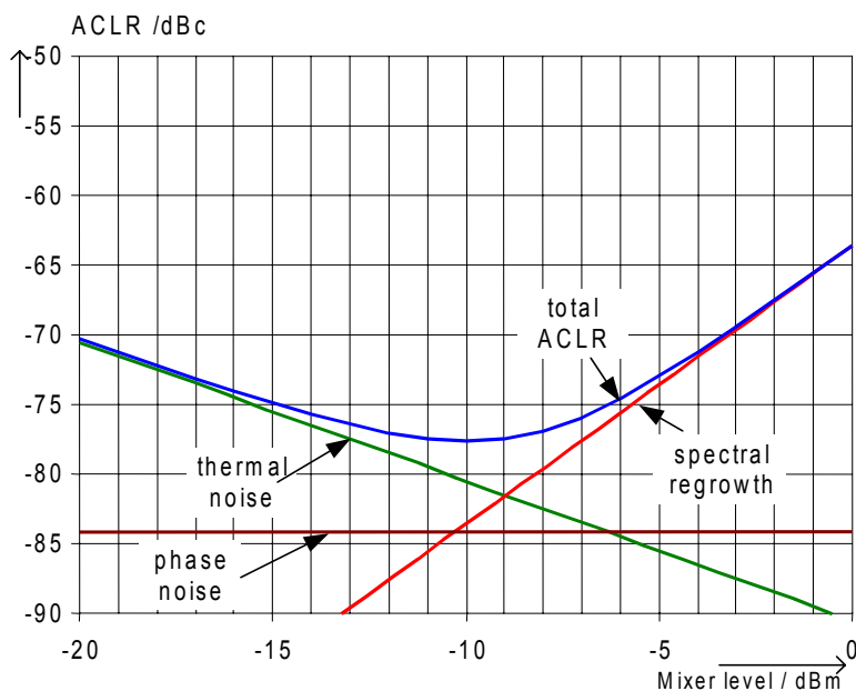
Bild 2-34 Dynamik des R&S FSQ bei Nachbarkanalleistungsmessung an W-CDMA-Uplink-Signalen abhängig vom Mischerpegel.
