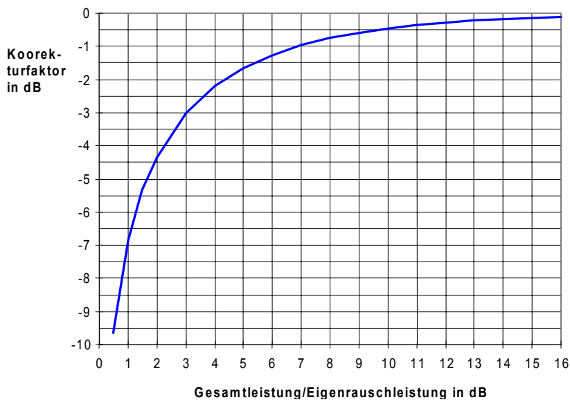
Bild 2-13 Korrekturfaktor für die gemessene Rauschleistung abhängig von Abstand zu Eigenrauschleistung des Signalanalysators
