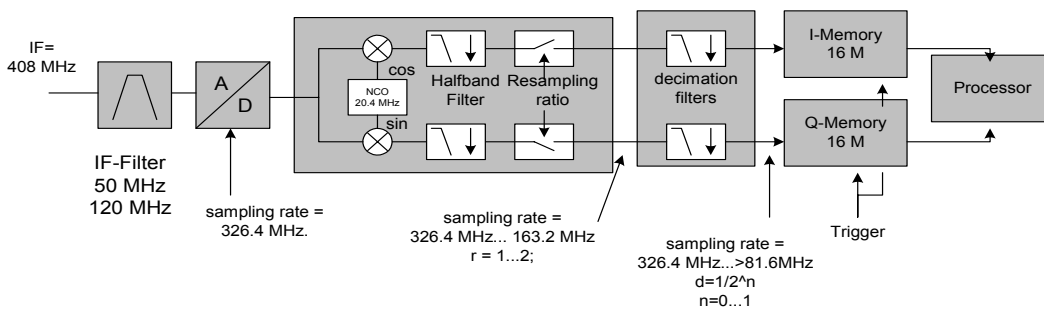
Bild 6-2 Blockschaltbild mit der Signalverarbeitung des R&S FSQ bei Abtastraten > 81.6 MHz
