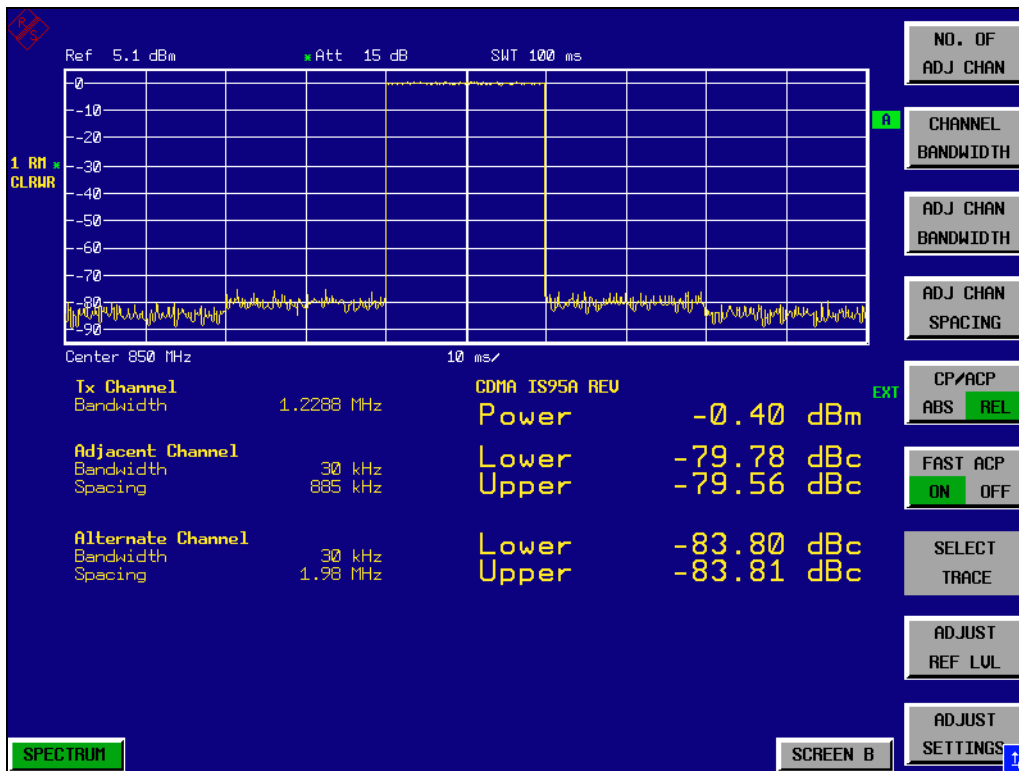
Bild 2-24 Messung der Kanalleistung und des Nachbarkanalleistungsabstandes bei IS95-Signalen im Zeitbereich (Fast ACP)
